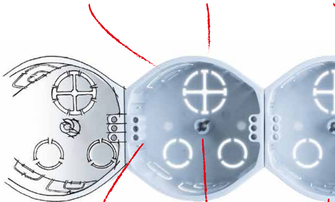
INTRĂRI COMBinate PENTRU TUBURI SI CABLURI
